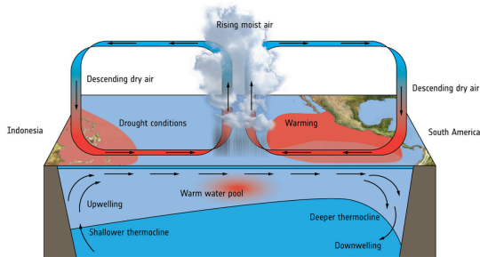
El Niño conditions
